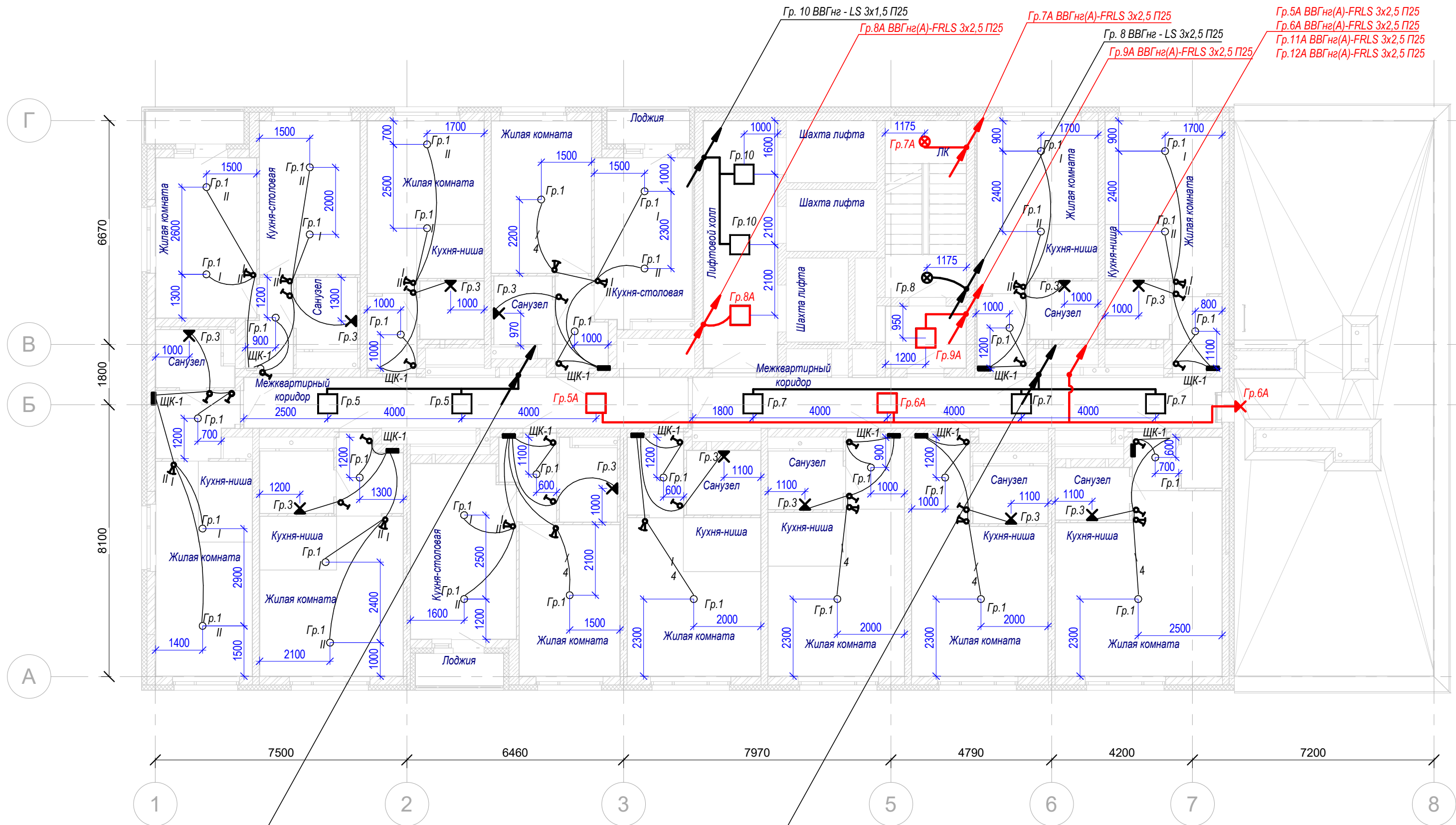
Планировка квартир на 26-27 этаже
